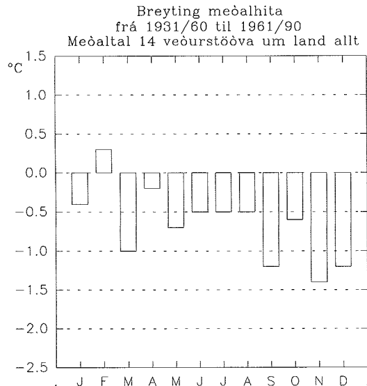
Mynd 1 / Fig. 1. Breyting meðalhita frá 1931/1960 til 1961/1990. Meðaltal 14 veðurstöðva í öllum landshlutum. Temperature change 1931/1960 to 1961/1990, an average of 14 stations around the country.
